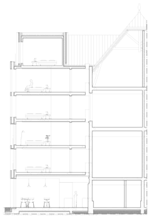
Querschnitt, neues und altes Gebäude
