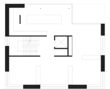
Grundriss Gartenniveau
