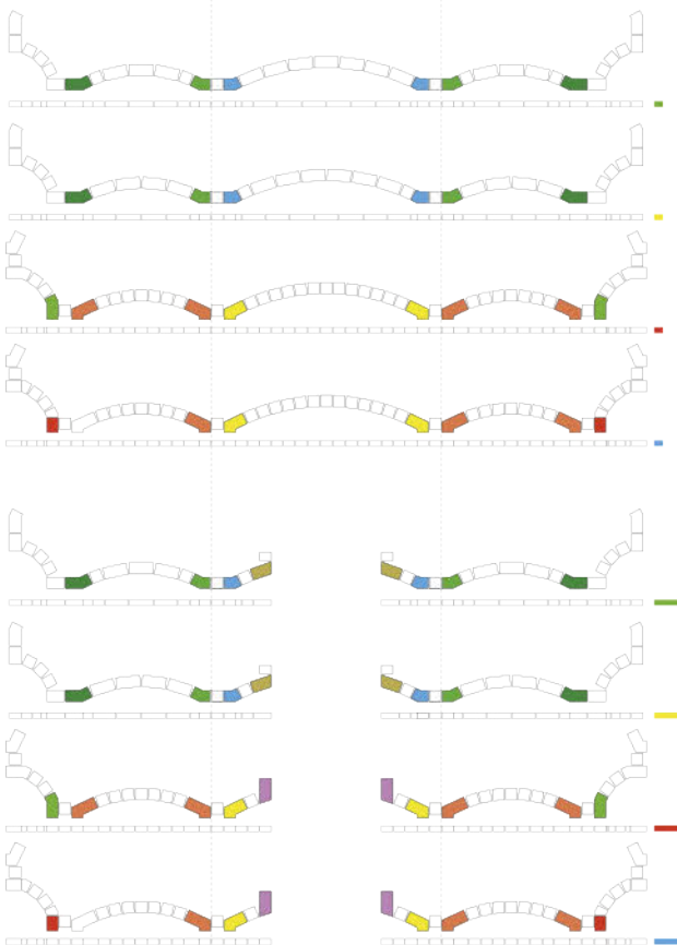
Aufsichten des Mauerverbands mit Spezialsteinen
