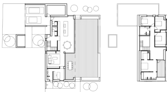
Grundriss Erdgeschoss
