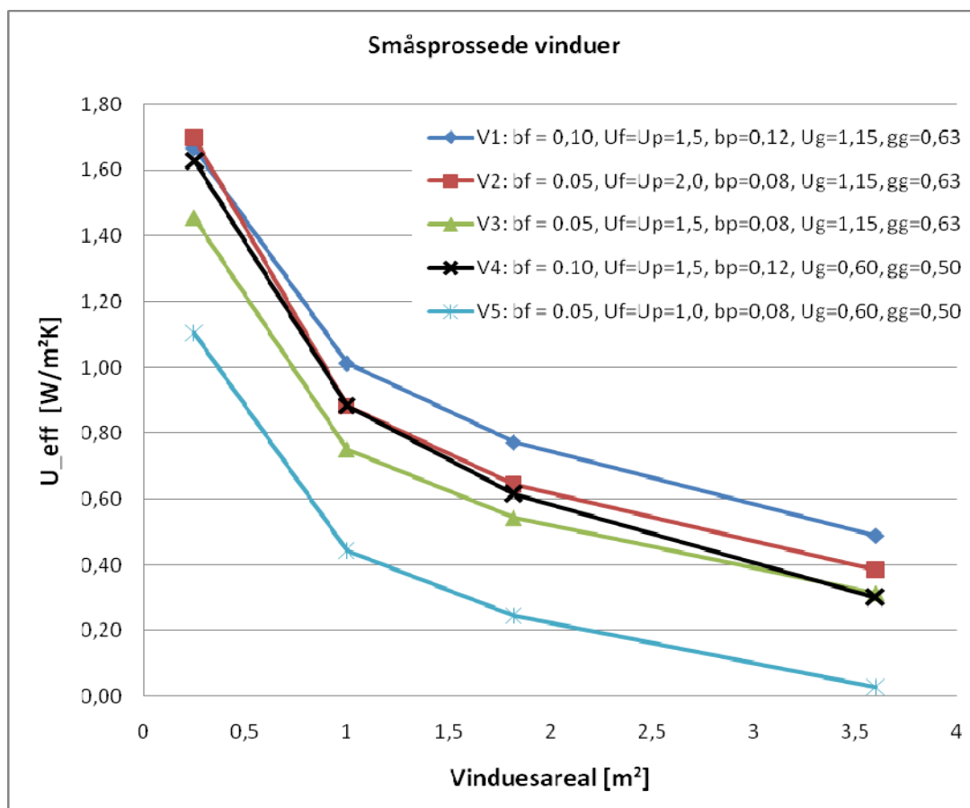
Figur 7. U_{eff} som funktion af vinduesstørrelsen for 5 forskellige småsprossede vinduer.
