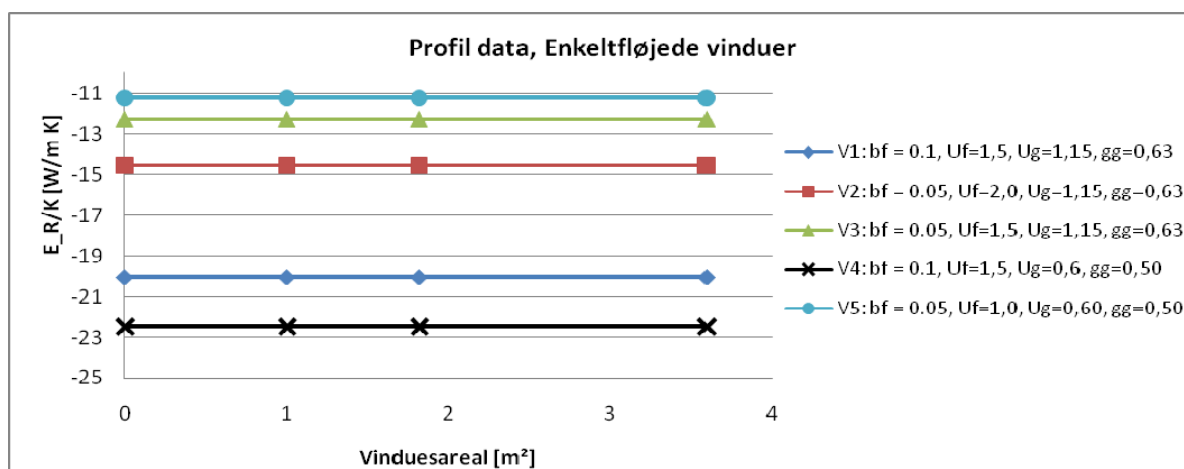
Figur 8. Energitilskud for ramme/karmprofiler for enkeltfløjede vinduer i forskellige størrelser.
