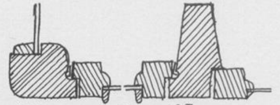
Hjørnevindue af træ © Sven Vedstrup 04
